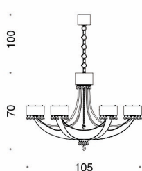
512/8 8 x G9 MAX 33W CE
